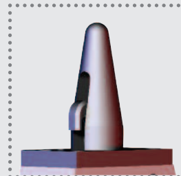
GPD30-530 Ø28.1 - Ø33.0
